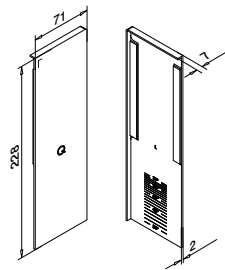
Links Für MOD 8234 Für Treppenmontage
