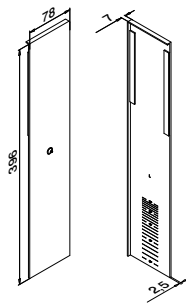
Links Für MOD 8444 Für Treppenmontage
