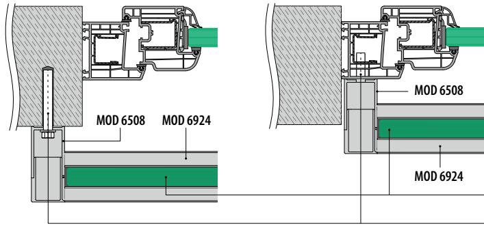
Fassadenmontage
