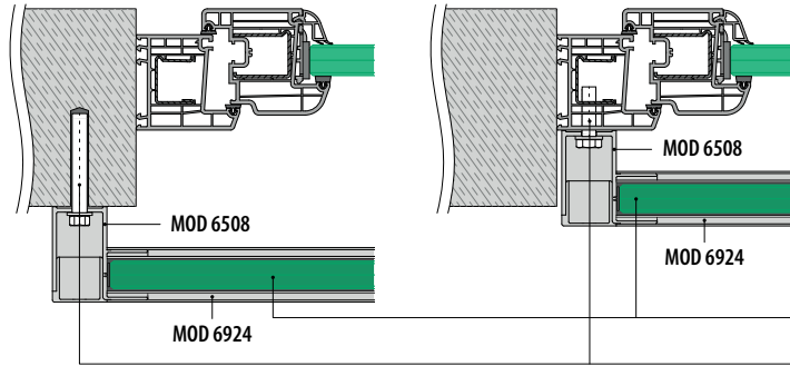
Fassadenmontage
