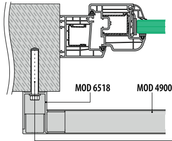
Fassadenmontage
