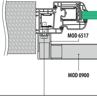
Rahmenmontage
