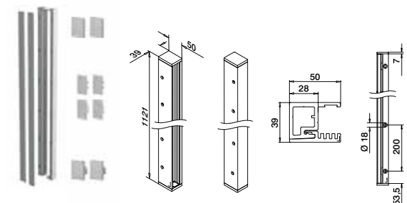
Fassaden- / Rahmenmontage
