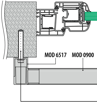
Fassadenmontage
