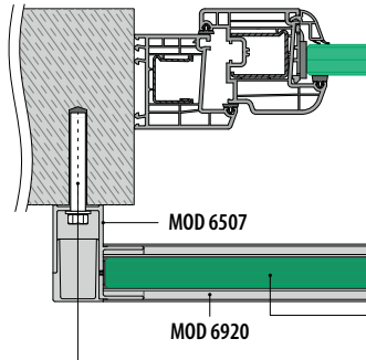
Fassadenmontage
