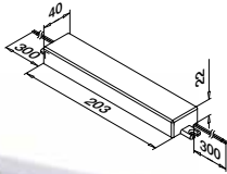
Transformator 12V 220...240V~, CE, ohne Stecker
