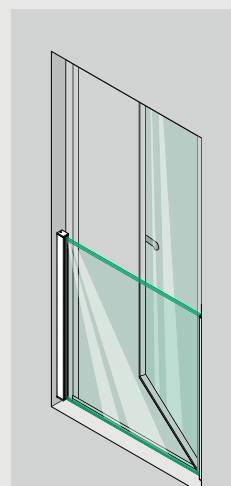
Montage in der Fensterlaibung
