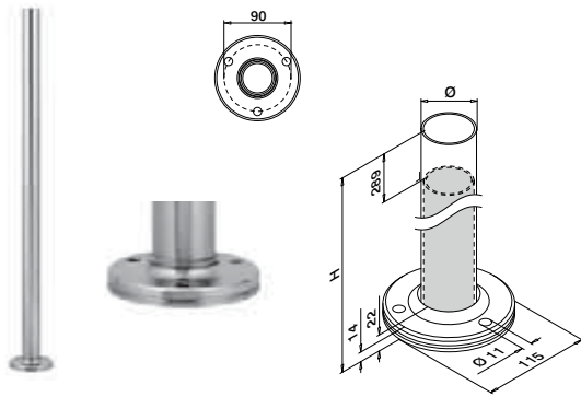
MOD 0916 - DOPPELTE WANDSTÄRKE 4,6 mm
