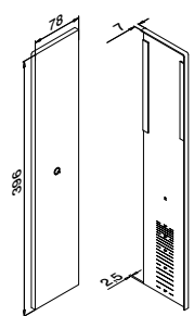
Rechts Für MOD 8444 Für Treppenmontage
