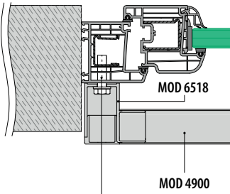
Rahmenmontage
