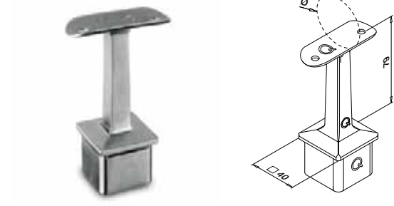
Für flaches Rohr zu rundem Rohr
