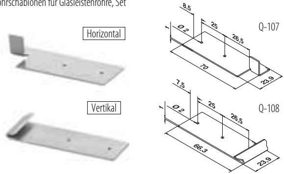
Bohrschablonen für Glasleistenrohre, Set
