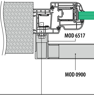
Rahmenmontage
