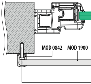
Fassadenmontage
