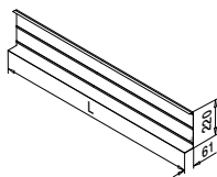
Blendleiste Vorderseite
