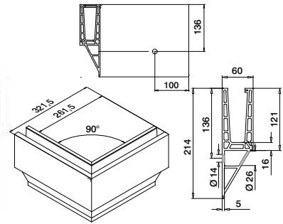
Aussenecke
