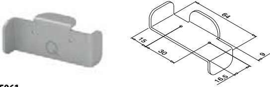
Bohrschablone für Easy Alu Geländerpfosten
