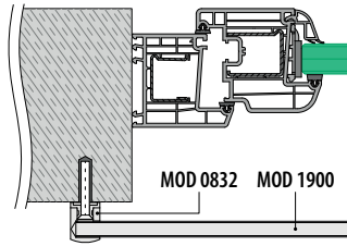
Fassadenmontage
