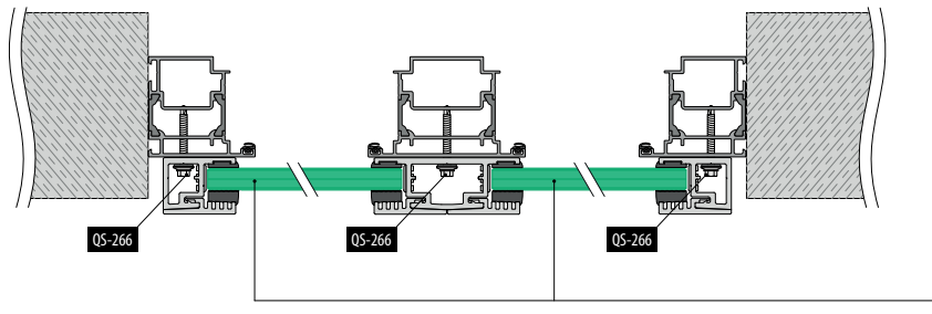
Montage mit Mittelprofil
