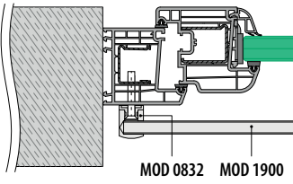
Rahmenmontage
