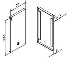
Links Für MOD 8234
