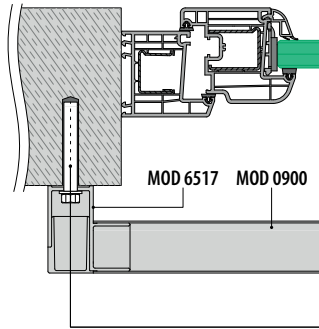
Fassadenmontage
