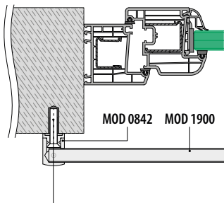
Montering på fasade
