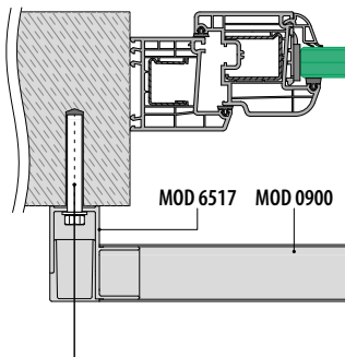
Montering på fasade
