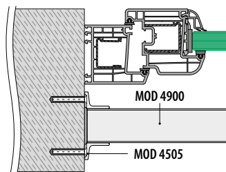
Montering i sidekantene
