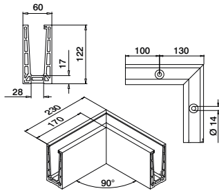
Innvendig hjørne
