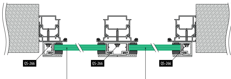
Montaż z profilem pośrednim
