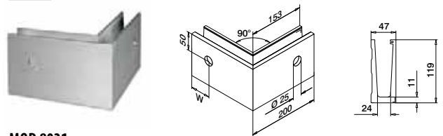
Narożnik zewnętrzny
