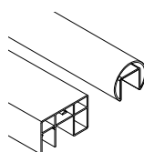
PROFILE NA SZKŁO / POCHWYT
