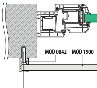
Montaż do fasady
