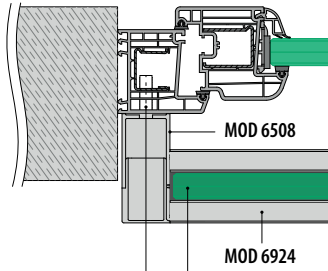
Montaż do ościeżnicy
