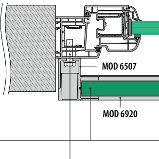
Montaż do ościeżnicy
