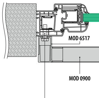
Montaż do ościeżnicy
