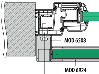
Montaż do ościeżnicy
