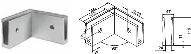
Narożnik wewnętrzny
