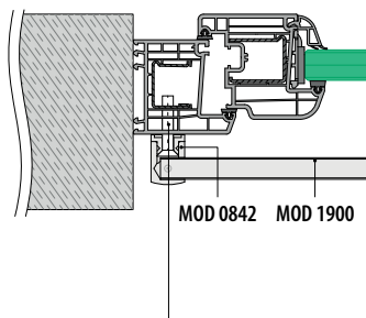
Montaż do ościeżnicy
