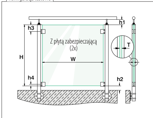
Konfiguracja testowa
