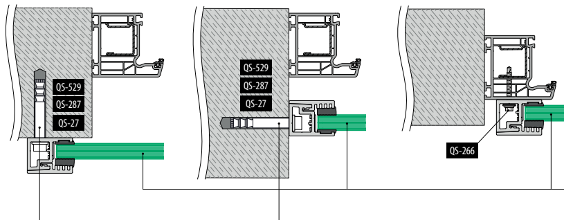
Montaż z profilem pośrednim
